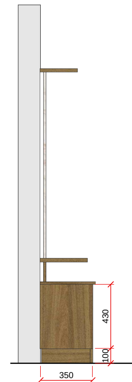
VISTA A - LATERAL - ESC. 1:25
